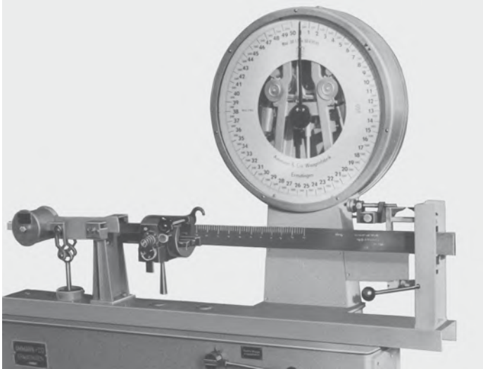
Waagbalken mit Billettdruckapparat und Kreiszeigerkopf
