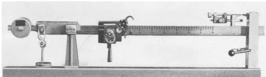
Waagbalken mit Billettdruckapparat
