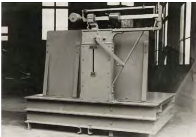
Mechanische Aufstellwaage mit Waagbalken
