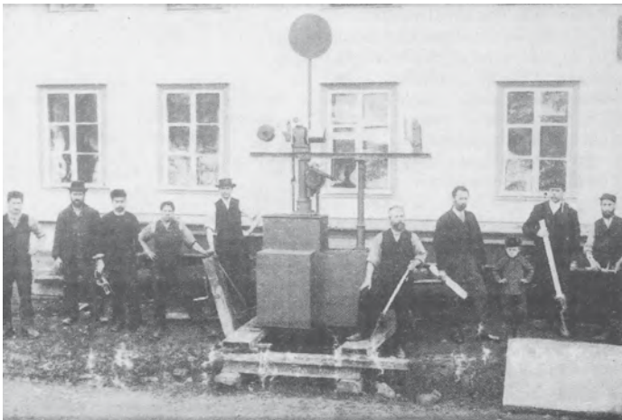
Justage einer Grosswaage um 1900
